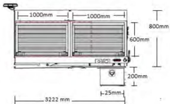
Vista izquierda estructura
