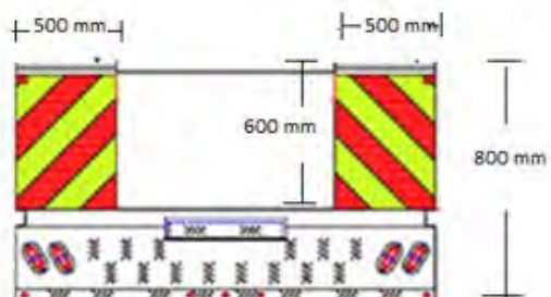
Vista posterior estructura
