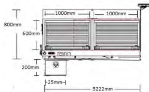
Vista derecha estructura
