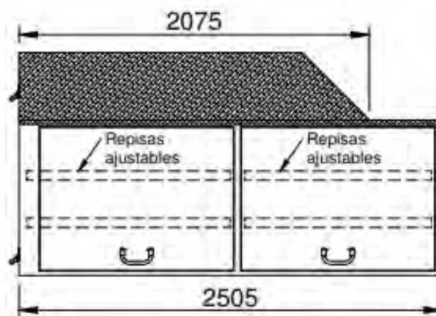
Vista derecha cúpula
