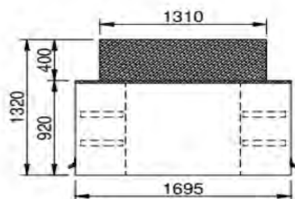
Vista frontal cúpula
