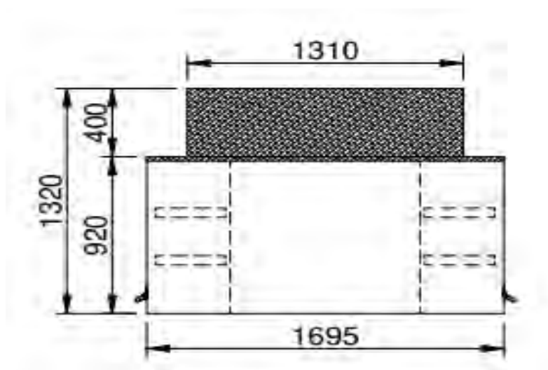
Vista frontal cúpula
