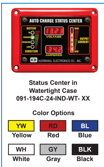
Status Center Display 091-194C-24-IND
